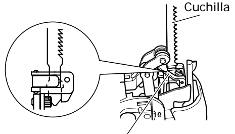
Portacuchilla
